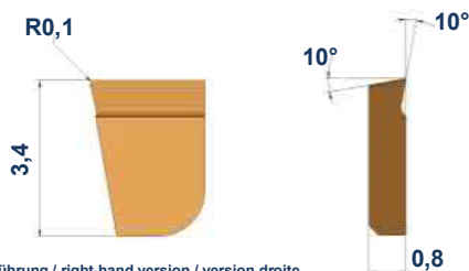
Rechtsausführung / right-hand version / version droite
