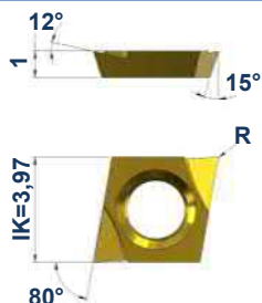
CDGT-0401...L
