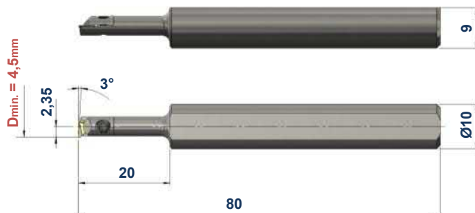
Rechtsausführung / right-hand version / version droite
