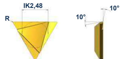
Linksausführung / left-hand version / version gauche
